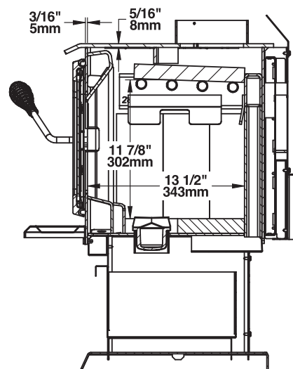
Chambre à combustion - Vue de côté
