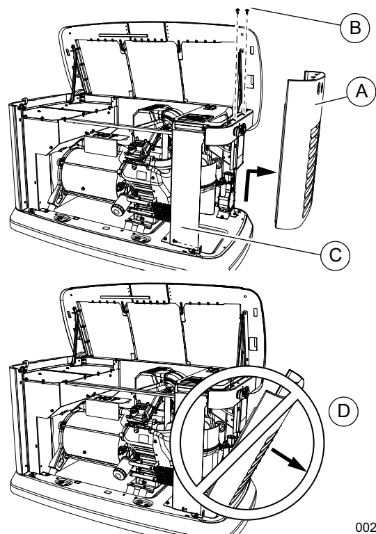
Figure 3-3. Dépose du panneau latéral d'admission
