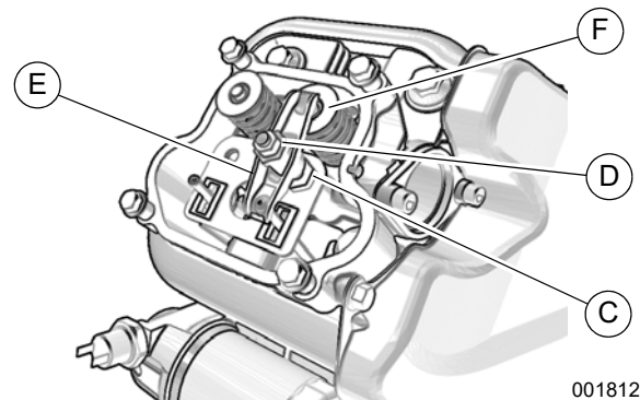
Figure 4-7. Réglage du jeu des soupapes (10 kW)
