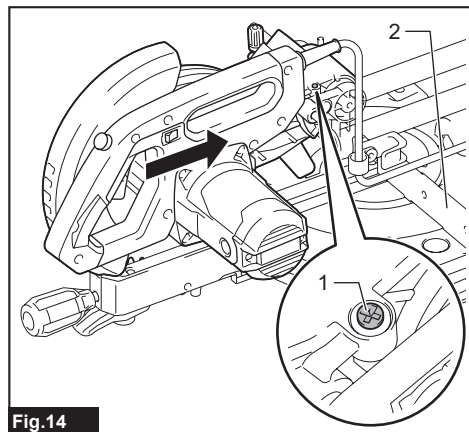
► 1. Boulon de réglage 2. Garde de guidage
