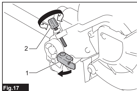
► 1. Bras de blocage 2. Vis de réglage
